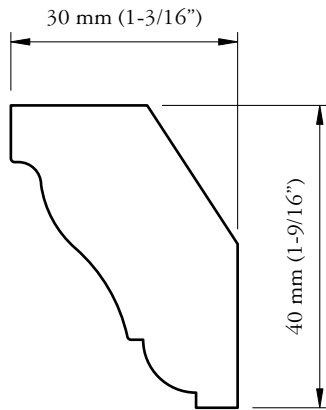
MC-30
