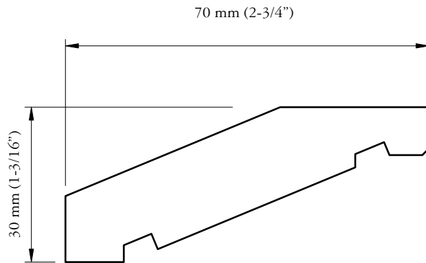
MC-90
